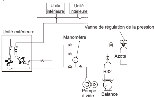
Fig.A Système de raccordement
